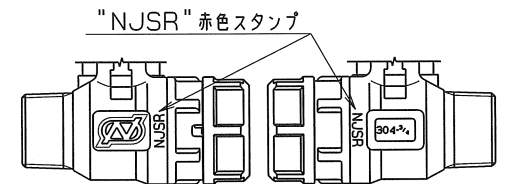
外觀図
